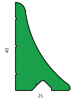
RD-40 weldorpel
